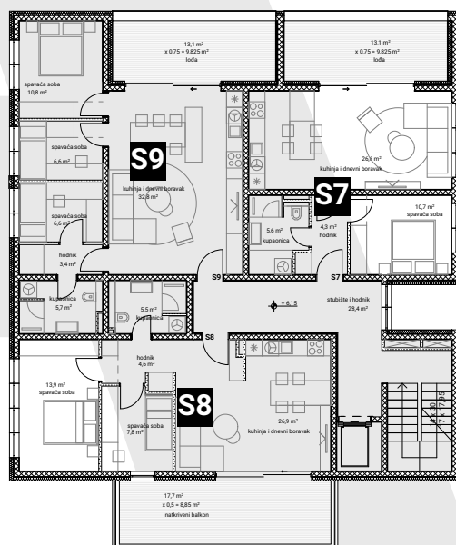
tlacrt 2. etaže
