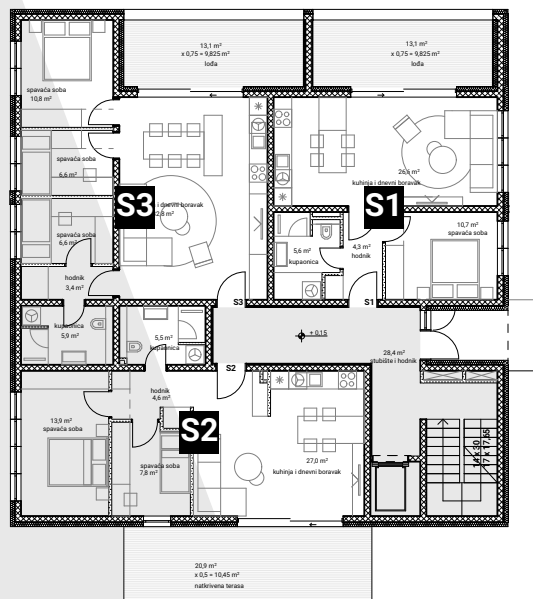
tlacrt prizemlja
